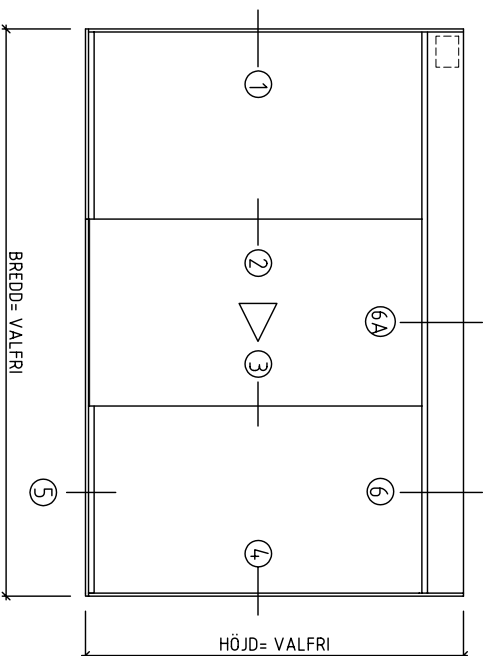
ELDIVEN SKJUTLUCKA TYP H80 RG 3- LUFT ALT A MÅTT 1500x1000. SEDD UTFRÅN SKALA 1:20 (A4) 2 FASTA PARTIER VID SIDORNA OCH ETT RÖRLIGT PARTI I MITTEN.
