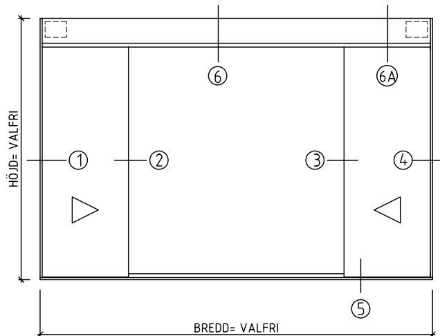
ELDRIVEN SKJUTLUCKA TYP H80 RG 3- LUFT ALT B MÅTT 1500x1000, SEDD UTFRÅN. SKALA 1:20 (A4). ETT FAST PARTI I MITTEN OCH TVÅ RÖRLIGA VID SIDORNA.
