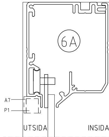
VERTIKALSNIITT 4A P1= UTFYLLNAD AV PROFIL, FYRKANTSPLAST 11x13 MM
