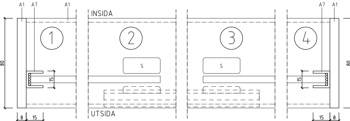
HORIZONTALSNITT STRECKADE LINJER VISAR FAST DEL. ▨ =CELLGUMMI, 2 MM
