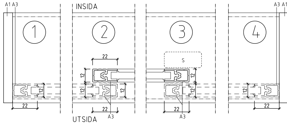
HORISONTALSNITT STRECKADE LINJER VISAR FAST DEL.
